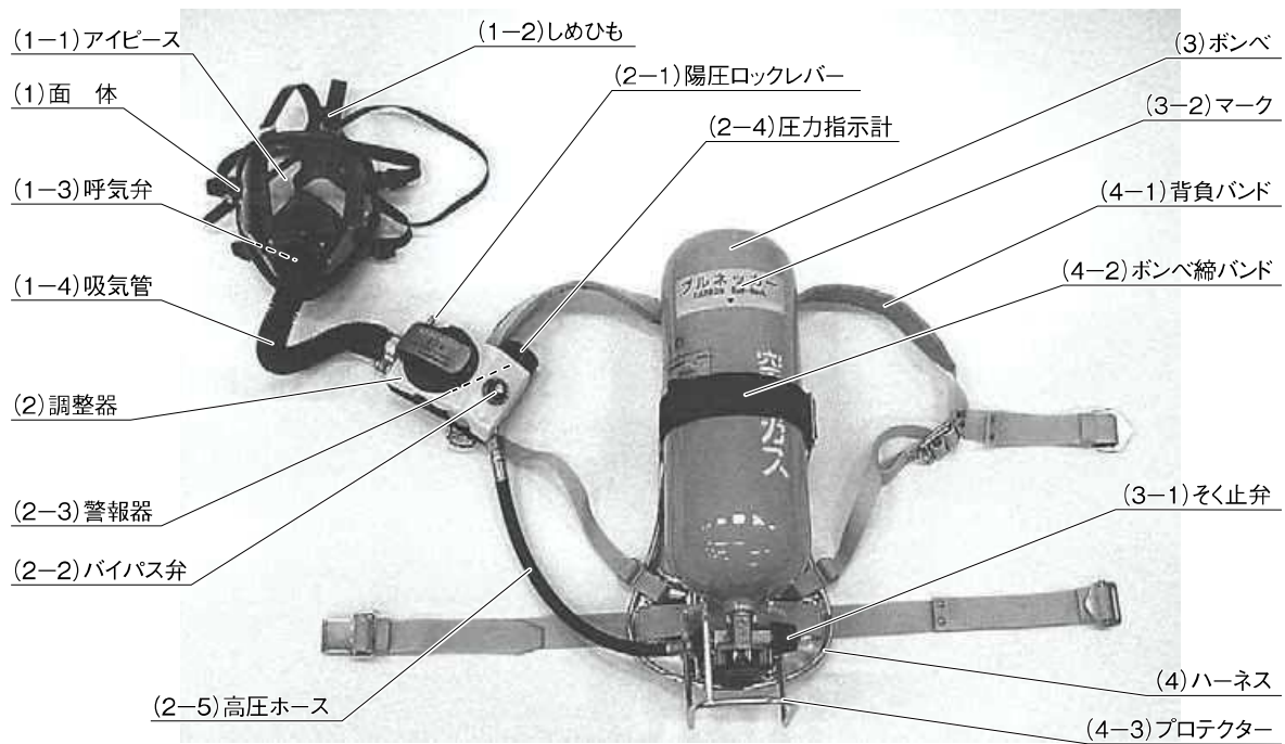
全体構成図
