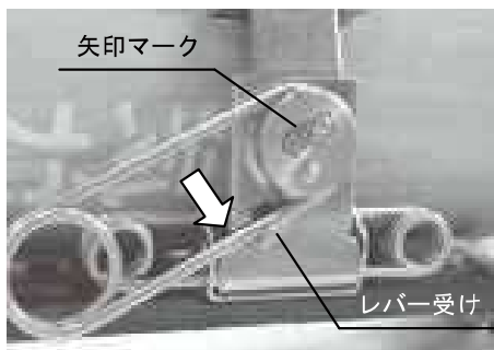
第6図 レバー受けにはめ込む
