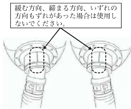
緩む方向のずれ 締まる方向のずれ 第11図 合いマークがずれている状態(例)
