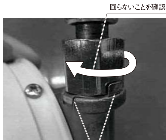
第15図 回り止め金具のつめ
