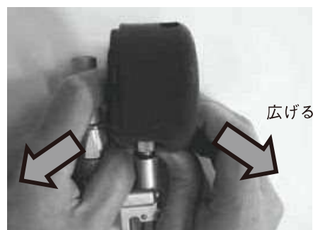
第25図 ゴムカバーを取り付ける
