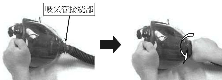
第12図 接続部のねじの緩み確認
