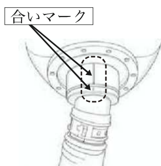
第10図 正しい位置 合いマークがずれていない状態
