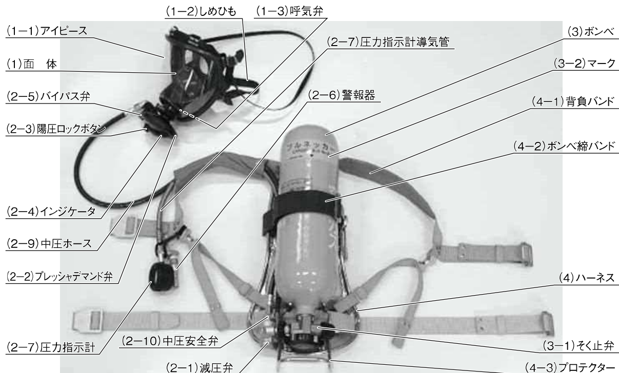
全体構成図
